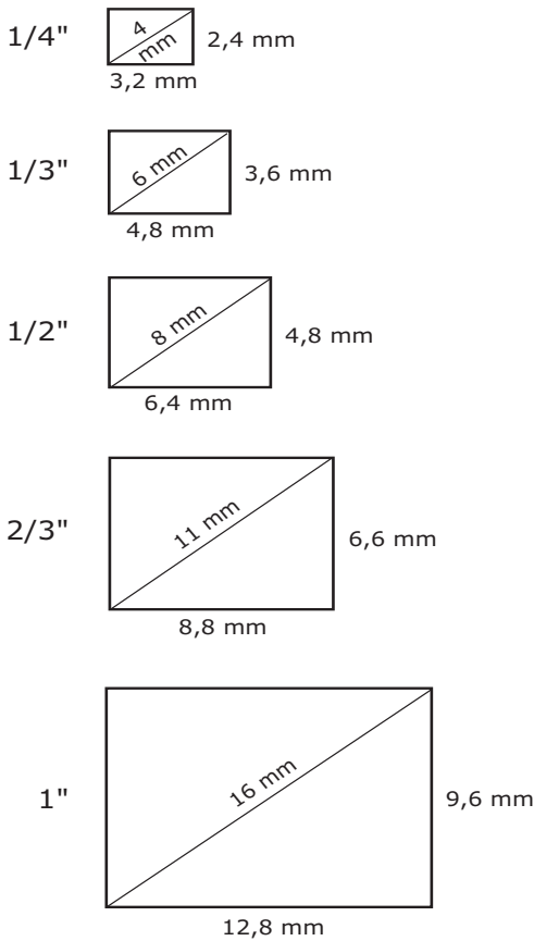
Fig. 2: CCD formats
